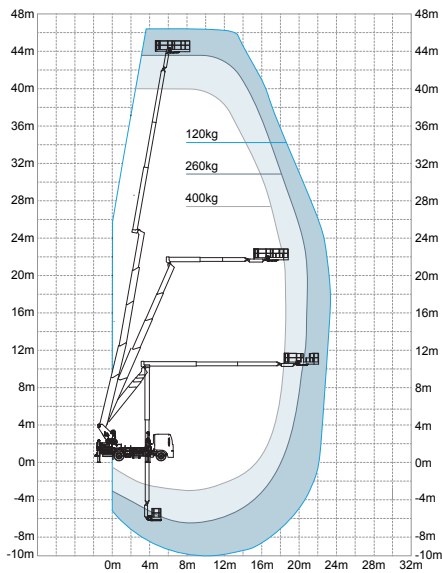
车头 0°~ 90°垂直作业曲线图
