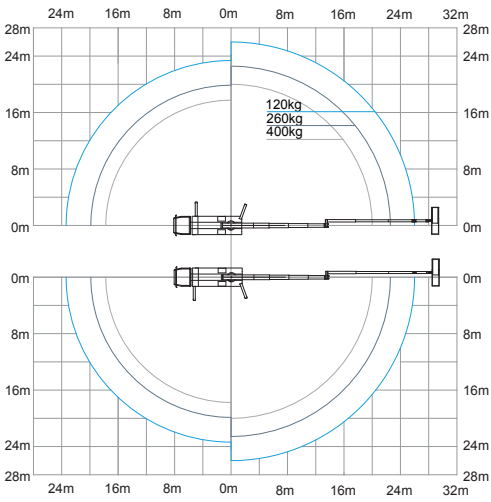
单边水平作业曲线图
