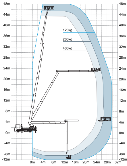
车后 151°~ 180°垂直作业曲线图
