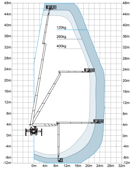
侧方 91°~ 150°垂直作业曲线图
