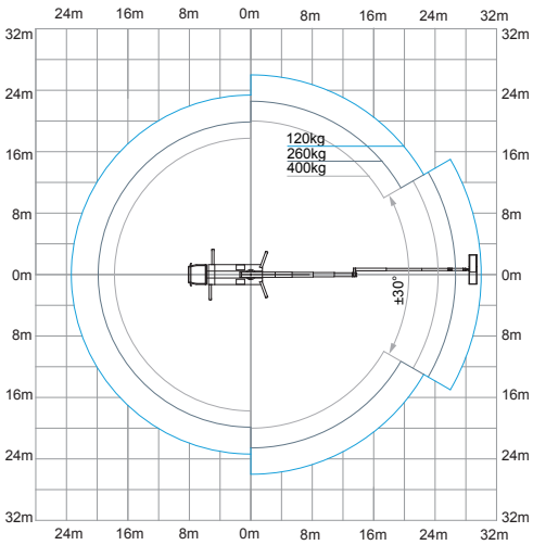
水平作业曲线图
